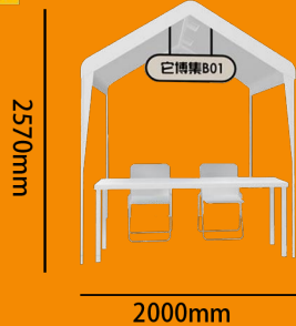
左视图
